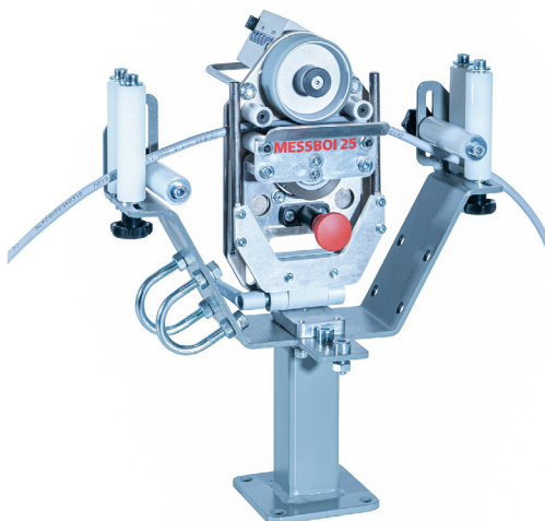
Abb. 2 MESSBOI 25 mit Rollenkäfigeinheit
