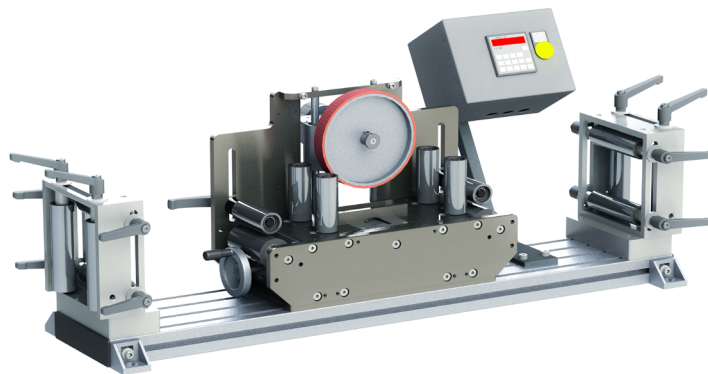
Abb. 1 MESSBOI 80 LC mit Gehäuse und Rollenkäfigen auf Aluprofil
