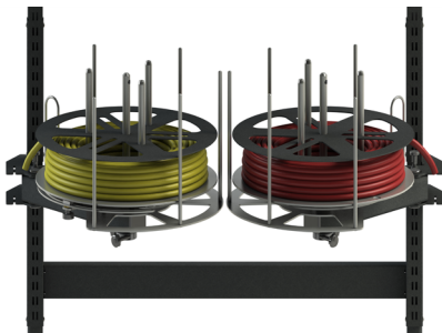
Abb. 13 MATBOI 480 T links / 480 T rechts mit Aufspringschutz beidseitig
