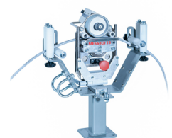
Abb. 3: MESSBOI 25 mit Rollenkäfigeinheit und Befestigungsvorrichtung
